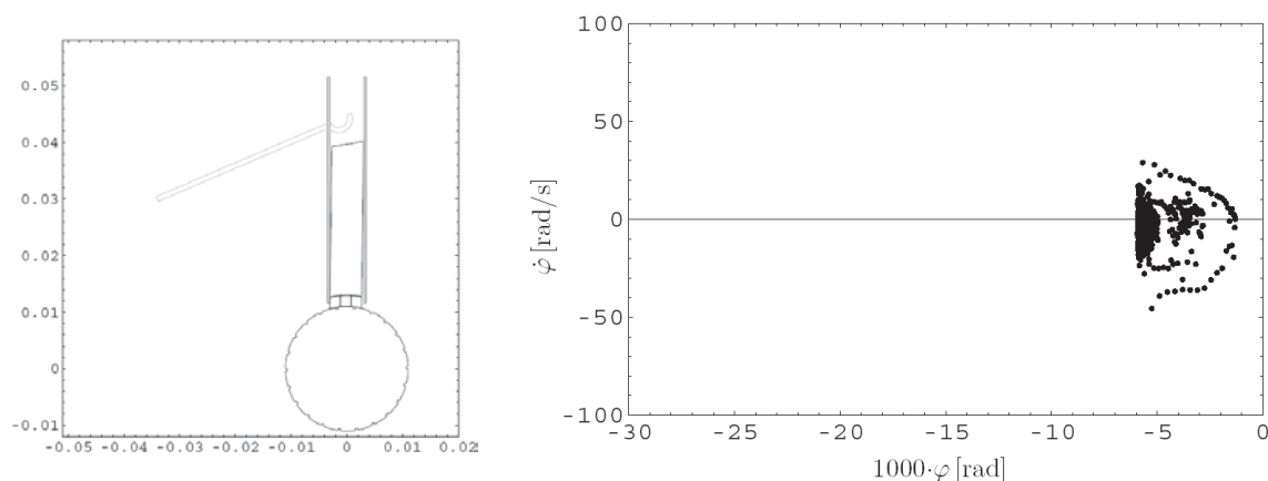
Sl. 5. Fazni diagram za \varphi pri novi ščetki Fig. 5. Phase diagram for \varphi for a new brush
