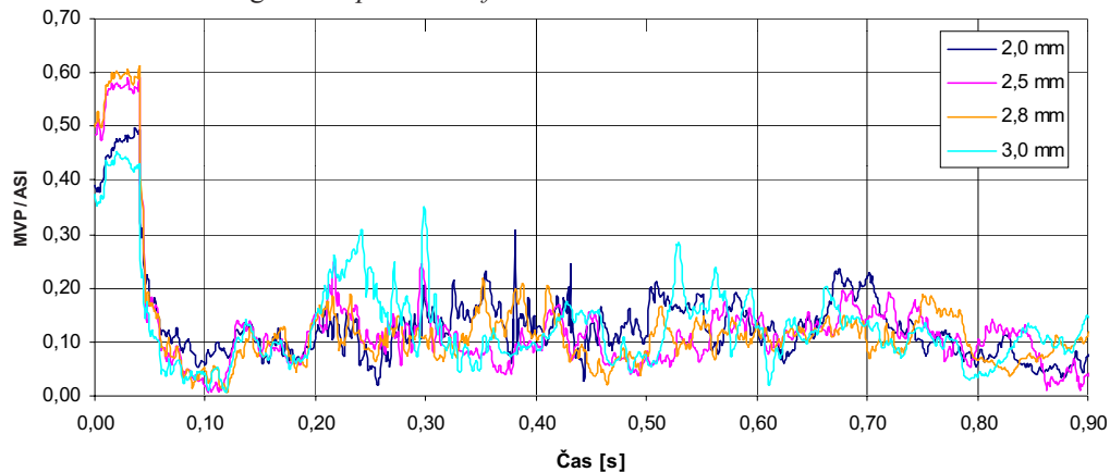
Sl. 9. Potek parametra MVP pri ograji z vodom
