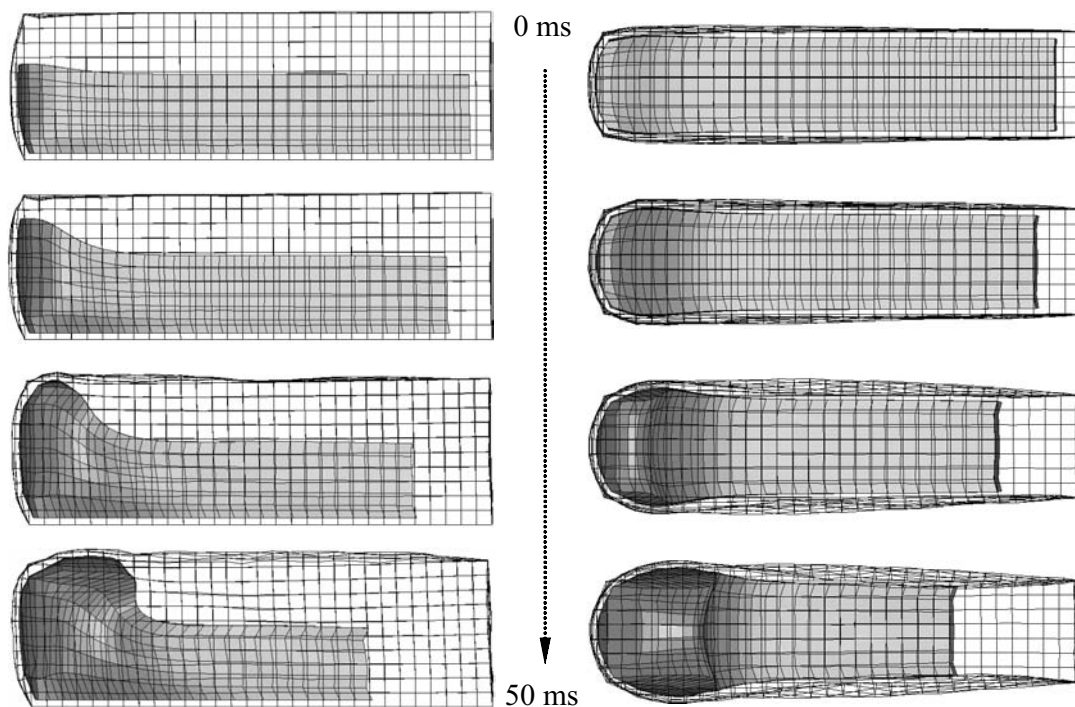
Sl. 12. Medsebojni vpliv tekočine in trdnine Fig. 12. Fluid-structure interaction
