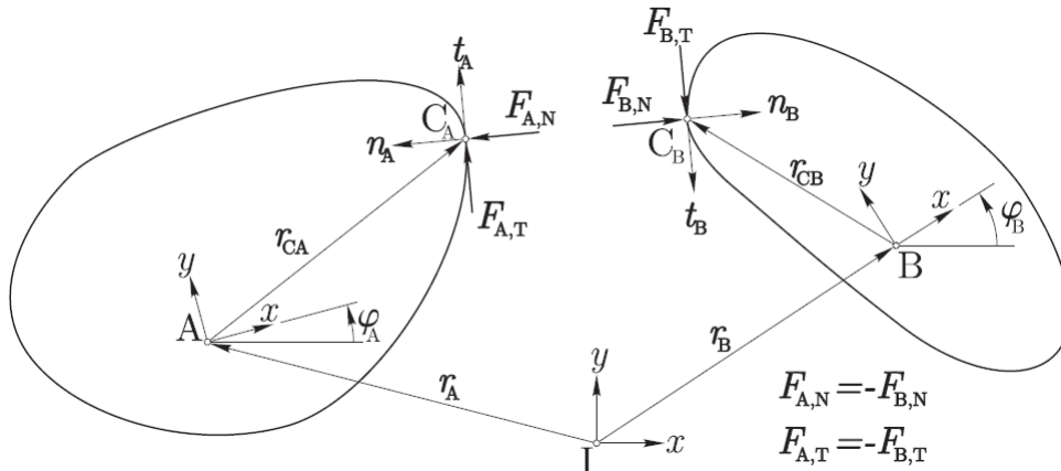
Sl. 1. Stične sile Fig. 1. Contact forces
