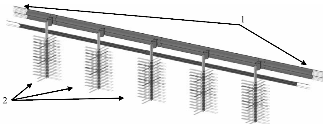
Sl. 5. Robni pogoji za varnostno ograjo s stebri, zabiti v zemljino
